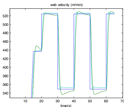
Fig. 9. Simulation results : web velocity
