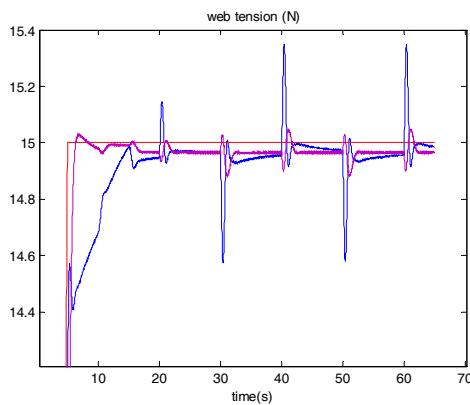
Fig. 8. Simulation results : web tension
